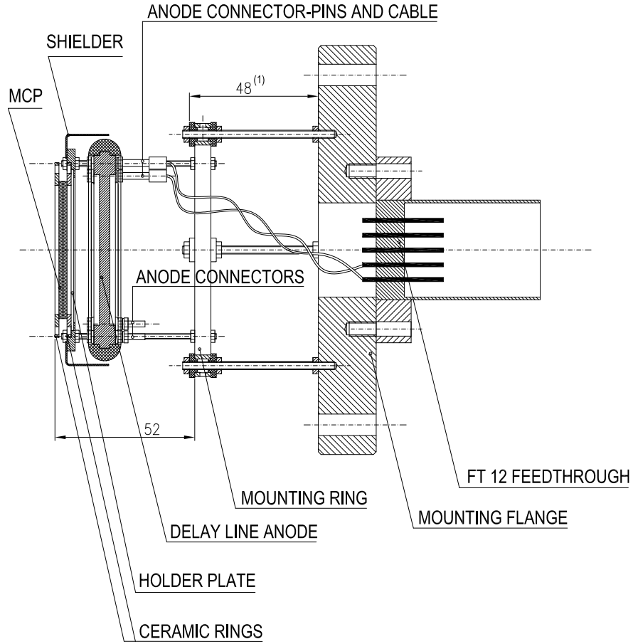
SECTION A-A
