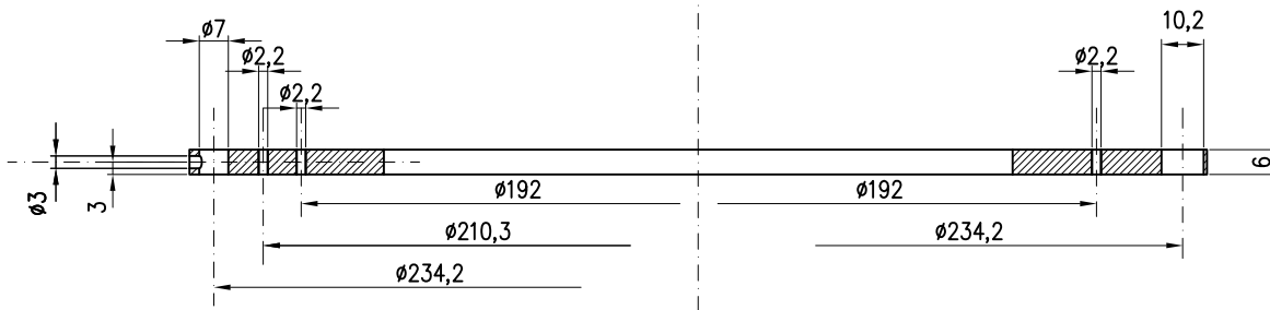
SCHNITT X-X
